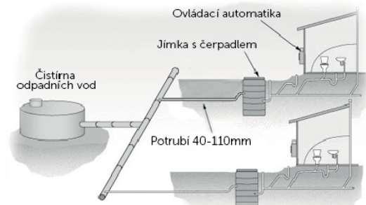
Schéma tlakové kanalizace.
